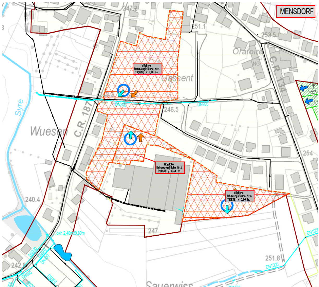
Abbildung 3 Darstellung der möglichen RW-Achsen sowie Vorplanung der Kanal- und MW-Behandlung
