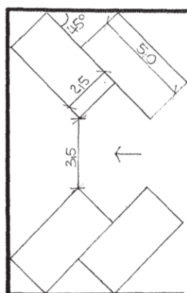
Figure 5 Dimensionnement des emplacements pour voitures
