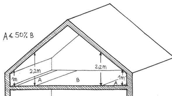
Figure 8 Hauteur libre sous plafond en cas d'une mezzanine ou de combles
