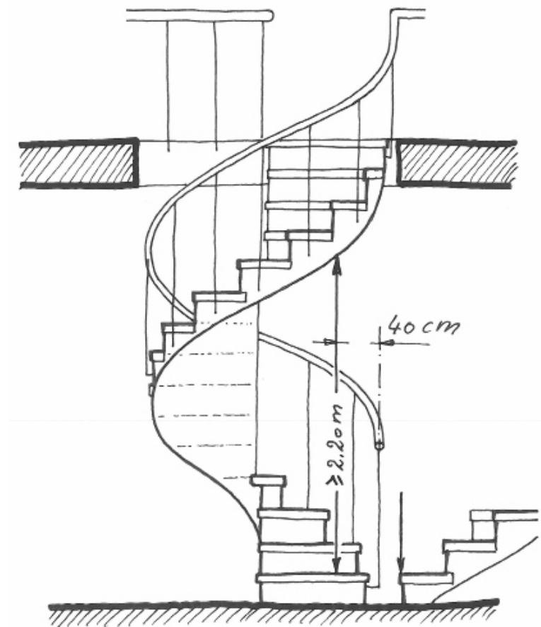
Figure 12 Géométrie d'un escalier en colimaçon ou à marches tournantes
