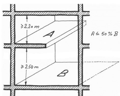
Figure 8 Hauteur libre sous plafond en cas d'une mezzanine ou de combles
