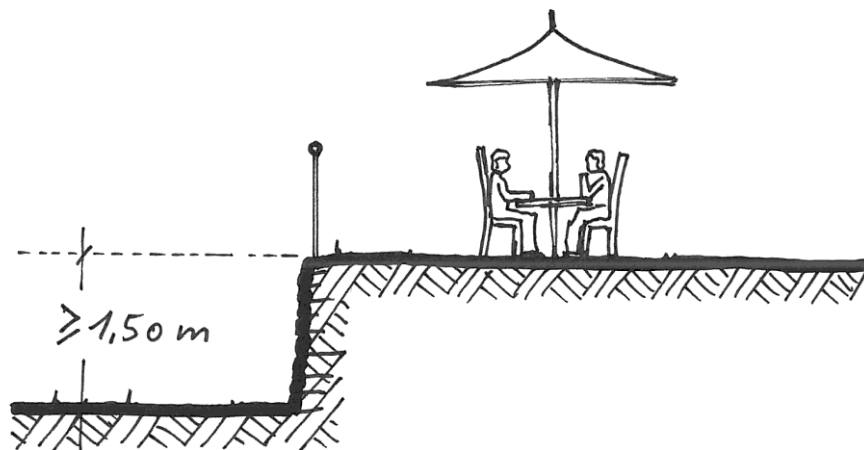
Figure 4 Garde-corps dans les aménagements extérieurs
